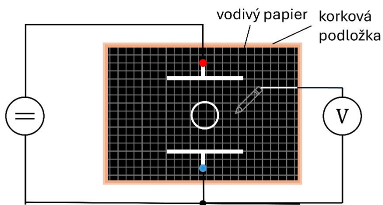
Obr. 10. Schéma zapojenia pre mapovanie elektrostatičného poľa v okolí vodivej uzavretej krivky umiestnenej medzi rovinnými elektródami
