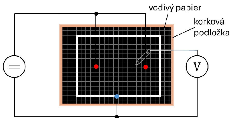
Obr. 9. Schéma zapojenia pre mapovanie elektrostatičného poľa v okolí dvoch súhlasne nabitých bodových nábojov
