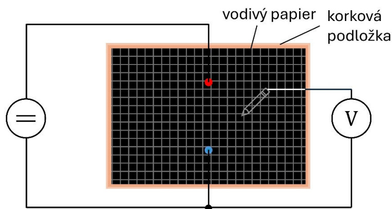
Obr. 8. Schéma zapojenia pre mapovanie elektrostatického poľa v okolí dipólu
