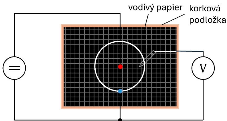
Obr. 7. Schéma zapojenia pre mapovanie elektrostatického poľa v okolí bodového náboj, ktorý sa nachádza vo vnútri plochy ohraničenej vodivou uzavretou krivkou
