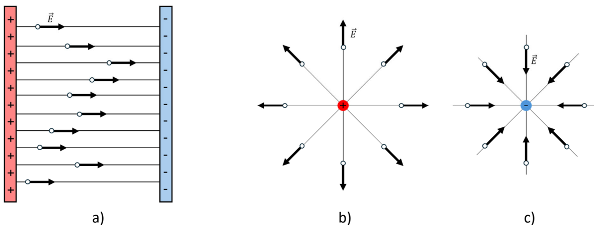
Obr. 3. a) Homogénne elektrické pole, b) Radiálne elektrické pole kladného náboja, c) radiálne elektrické pole záporného náboja
