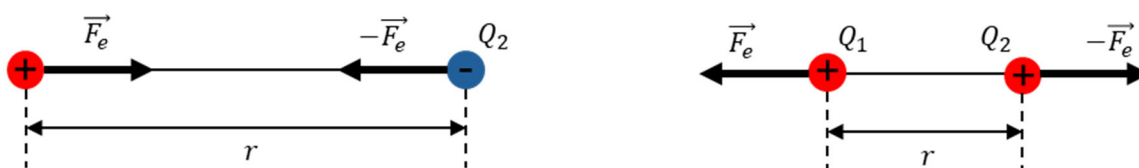
Obr. 1. Vzájomné silové pôsobenie medzi bodovými elektrickými nábojmi
