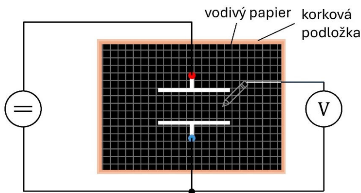
Obr. 13. Schéma zapojenia pre mapovanie elektrostatického poľa medzi dvomi paralelnými elektródami
