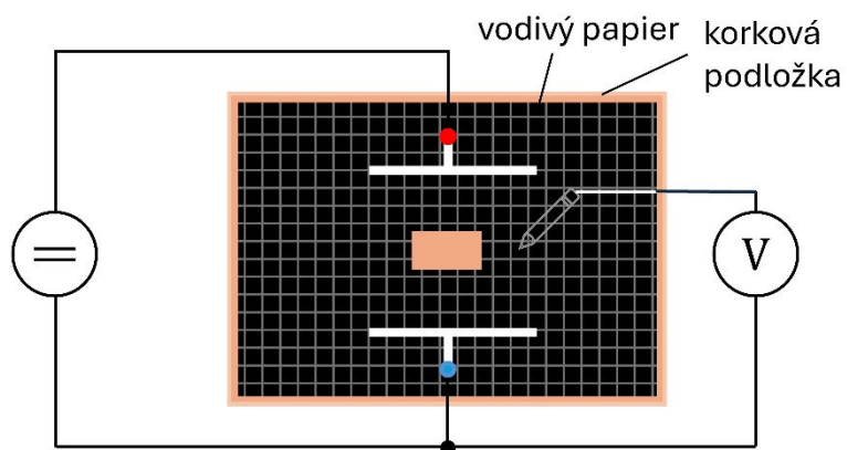
Obr. 11. Schéma zapojenia pre mapovanie elektrostatičného poľa v okolí obdĺžnikového izolátora umiestneného medzi rovinnými elektródami
