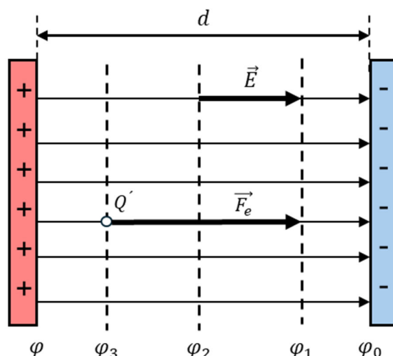
Obr. 6. Ekvipotenciálne plochy homogénneho elektrického poľa
