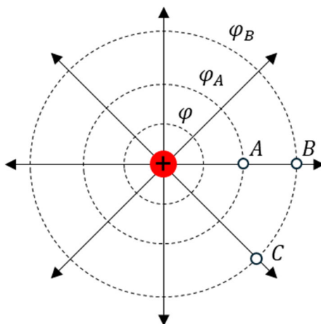
Obr. 5. Ekvipotenciálne plochy radiálneho elektrického poľa
